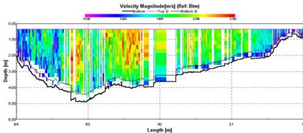
Obrázek 2 - Výstup z měření ADCP ve Vranově nad Dyjí.
