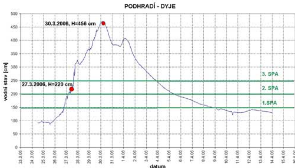
Obrázek 4 - Čára vodních stavů z vodoměrné stanice Podhradí nad Dyjí.
