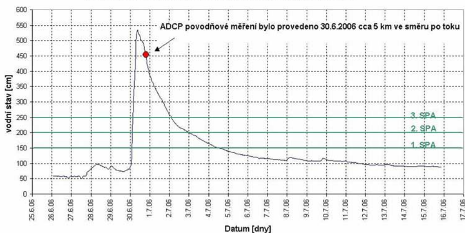
Graf 1 - Čára vodních stavů - vodoměrná stanice Podhradí nad Dyjí
